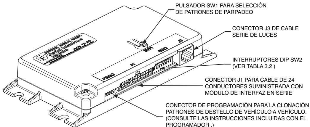
Figura 3.2: Módulo de interfaz en serie
