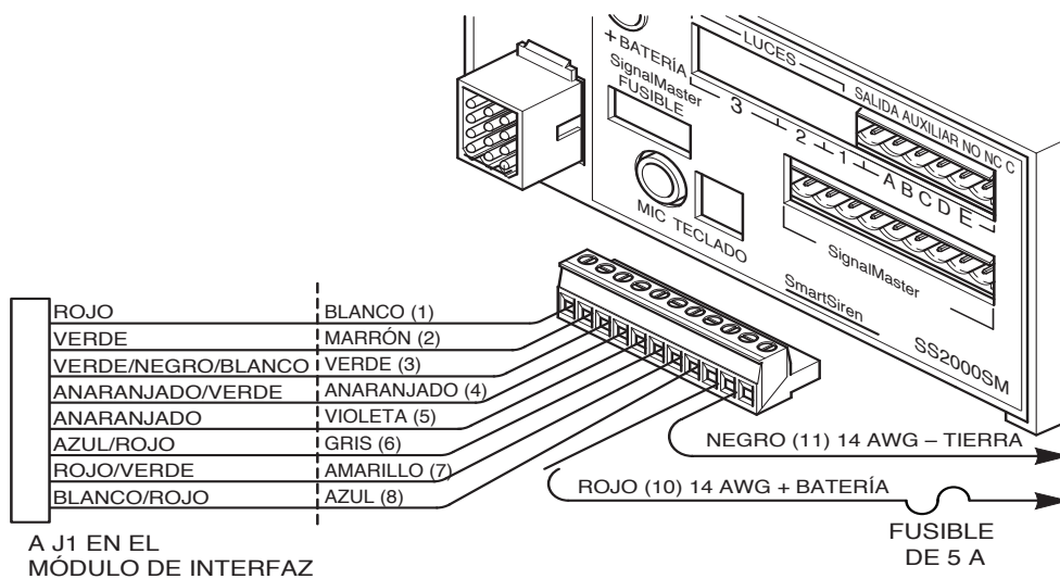
Figura 4.4: Controlador SmartSiren serie SS2000SM (externo)
