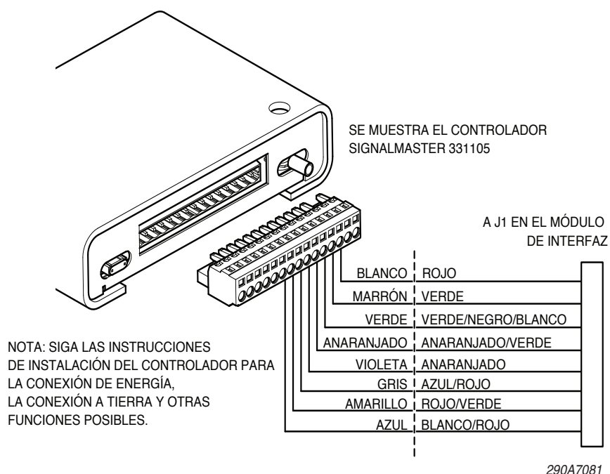
Figura 4.3: Controlador SignalMaster 331105 (externo)
