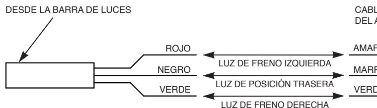
Figura 4.7: Cableado de las luces de freno/giro/cola trasera entre la barra de luces y el arnés del vehículo
