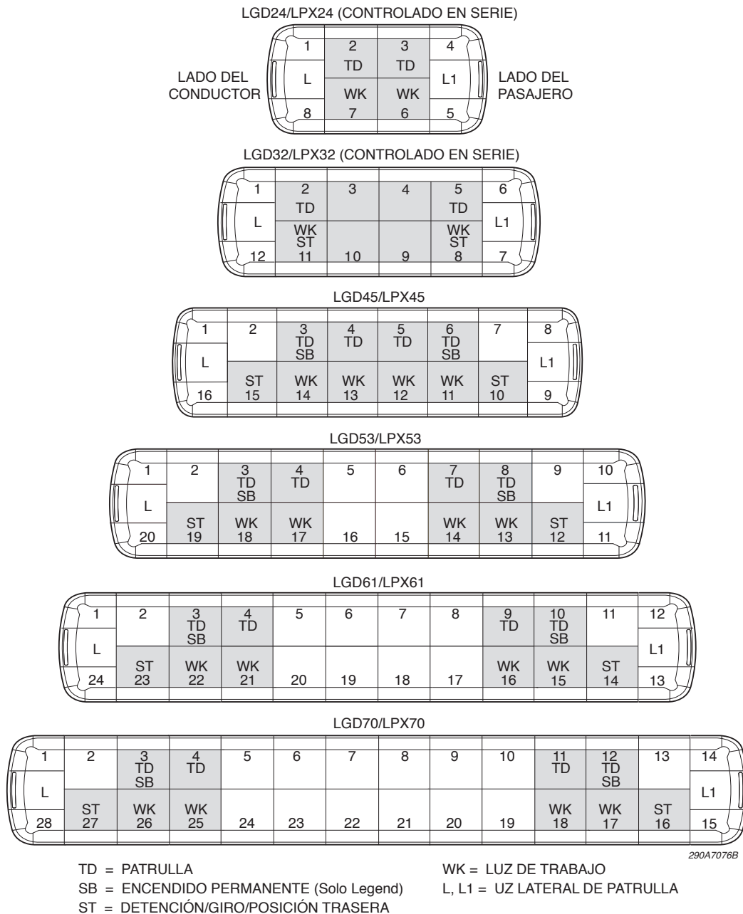
Figura 3.3: Opciones de luces para las barras de luces Legend
