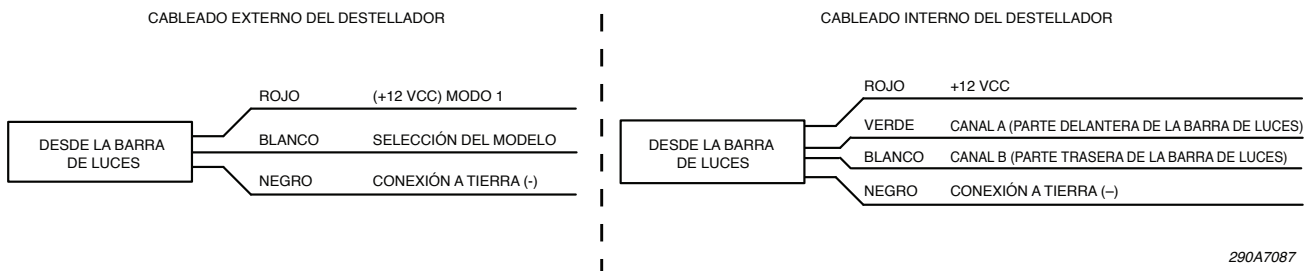
Figura 4.9: Conexión del destellador interno/externo para los productos Legend de 12 pulgadas
