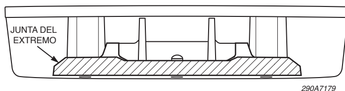
Figura 5.5: Junta del extremo en la cavidad de la base del extremo
