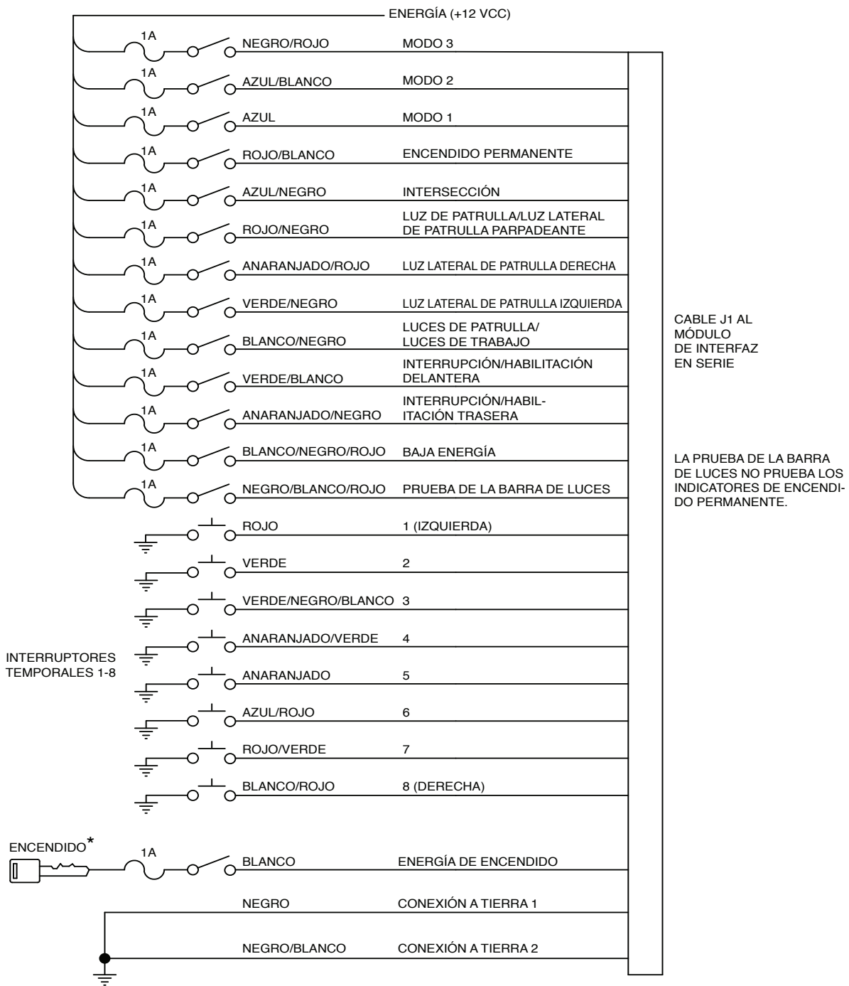
Figura 4.6: Funciones de control del SignalMaster conectadas a 12 VCC para control interno
